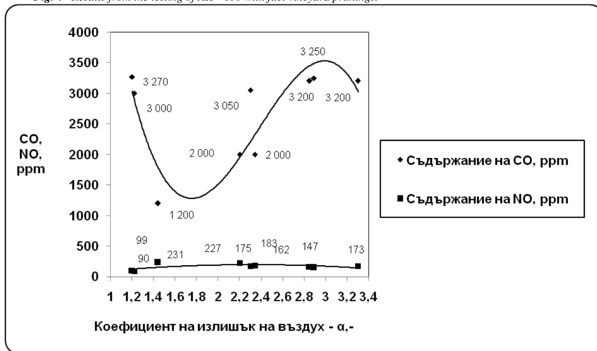
Фиг. 4 Резултати от изпитанието на ВП - 800 с гориво лозови пръчки. Fig. 4 Results from the testing of AH - 800 with fuel vineyard prunings.
