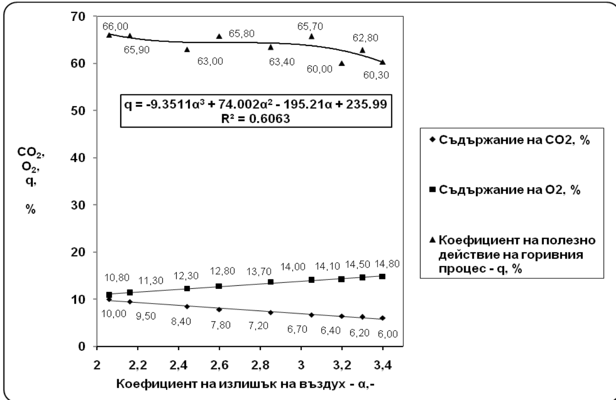
Фиг. 6 Резултати от изпитанието на ВП - 800 с гориво цепеници от тополя Fig. 6 Results from the testing of AH - 800 with fuel poplar logs.
