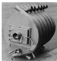
Фиг.1 Общ вид на ВП – 800 Fig.1 General view of AH - 800
