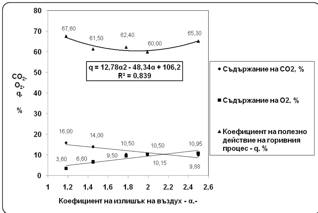
Фиг. 7 Резултати от изпитанието на ВП-800 с гориво клони от резитбата на ябълкови дървета Fig. 7 Results from the testing of AH - 800 with fuel branches from apple trees pruning
