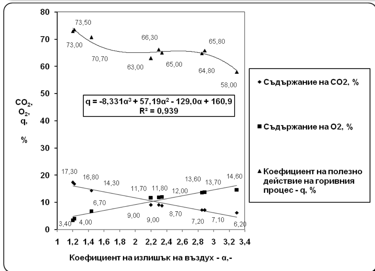
Фиг. 5 Резултати от изпитанието на ВП - 800 с гориво брикети от тютюнев прах. Fig. 5 Results from the testing of AH - 800 with fuel tobacco powder briquettes.
