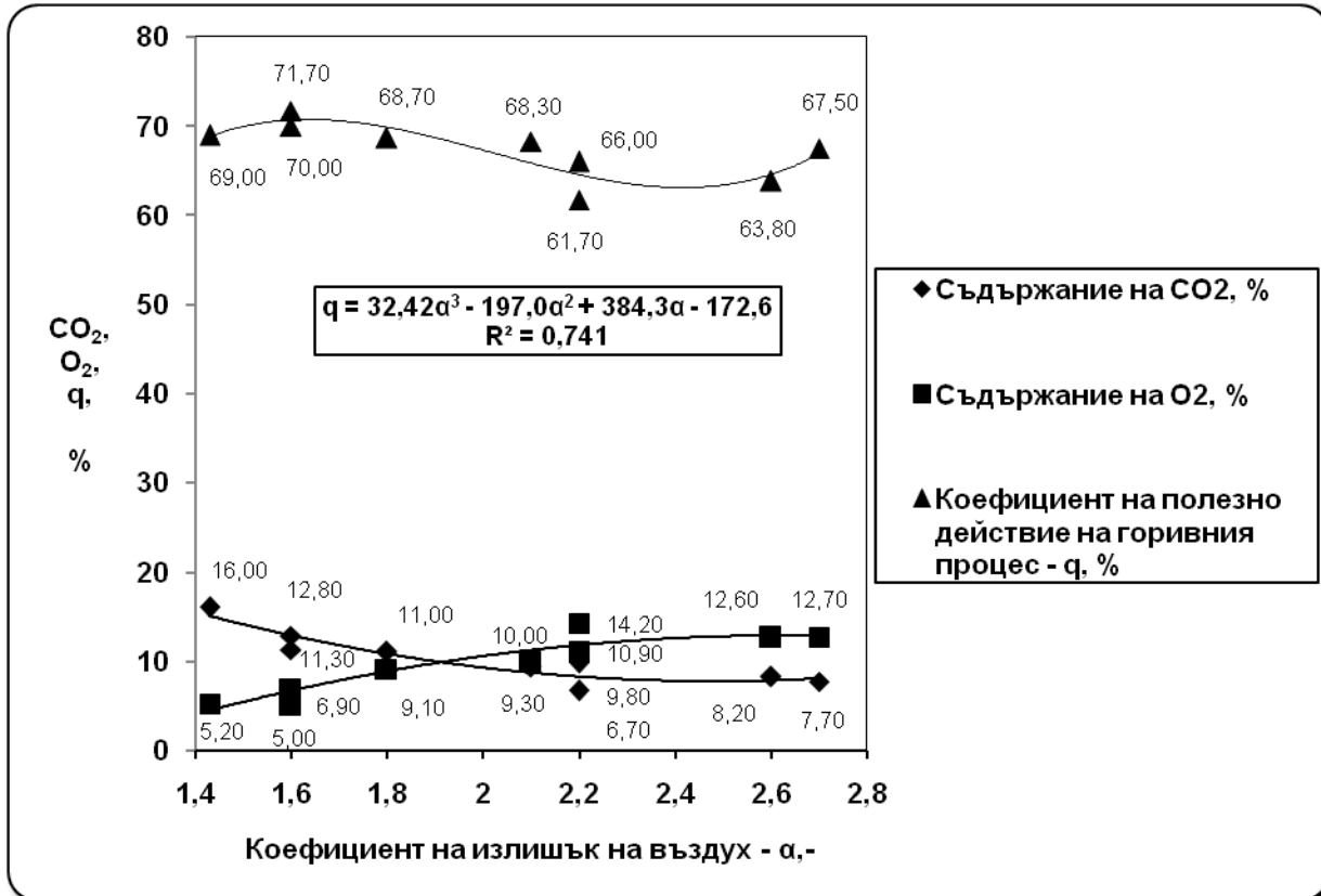
Фиг. 4 Резултати от изпитанието на ВП - 800 с гориво лозови пръчки. Fig. 4 Results from the testing of AH - 800 with fuel vineyard prunings.
